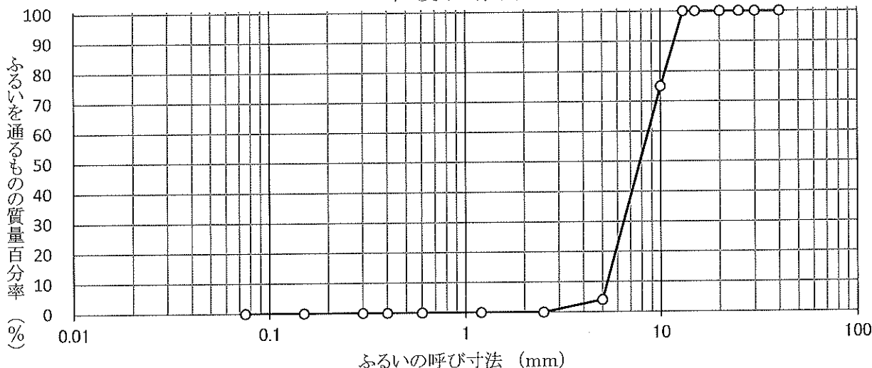
粒度曲線図
